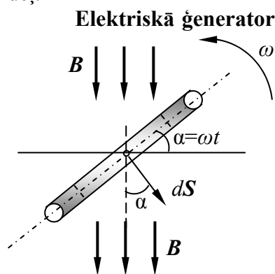
6.3. att. Ja spole rotē magnētiskajā laukā ar vienmērīgu leņķisko ātrumu \omega , tajā inducējas laikā sinusoidāli mainīgs EDS.
