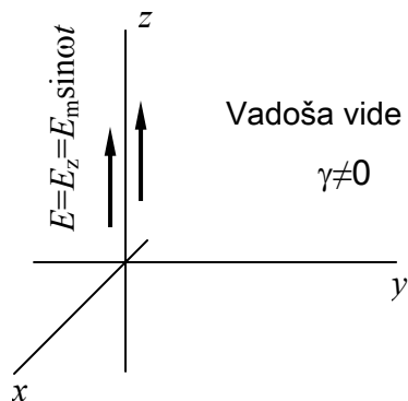
7.5. att. Uz x,z plaknes tiek uzturēta laikā sinusoidāli mainīga elektriskā lauka intensitāte. Kā izplatīsies viļņi vadošajā vidē?
