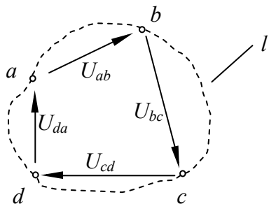
1.6. att. Spriegumu algebriska summa noslēgtā kontūrā ir vienāda ar 0.
