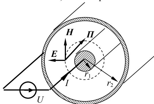
7.1. att. Telpā starp koaksiāla kabeļa vadiem \mathbf{E} vektors vērsts radiālā virzienā, \mathbf{H} – pa koncentriskā riņķa pieskari, bet \mathbf{\Pi} – aksiālā virzienā.
