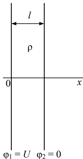
1.11. att. Plakana kondensatora matemātiskais modelis
