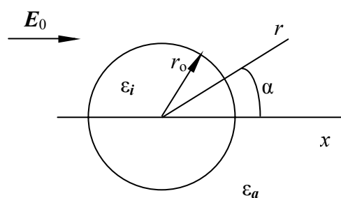
1.12. att. Garš cilindrs ārējā laukā. Potenciāls \varphi atkarīgs tikai no koordinātām r un \alpha cilindriskajā koordinātu sistēmā.
