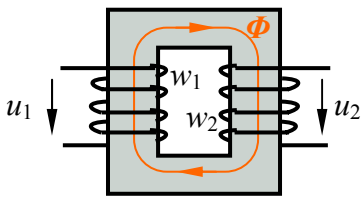
6.4. att. Transformatoru veido induktīvi saistītas spoles, novietotas uz kopējas noslēgtas feromagnētiska materiāla serdes.
