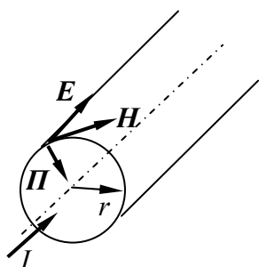
7.2. att. Enerģija, kas no apkārtējā elektromagnētiskā lauka ieplūst vadā, tiek patērēta vada silšanai.
